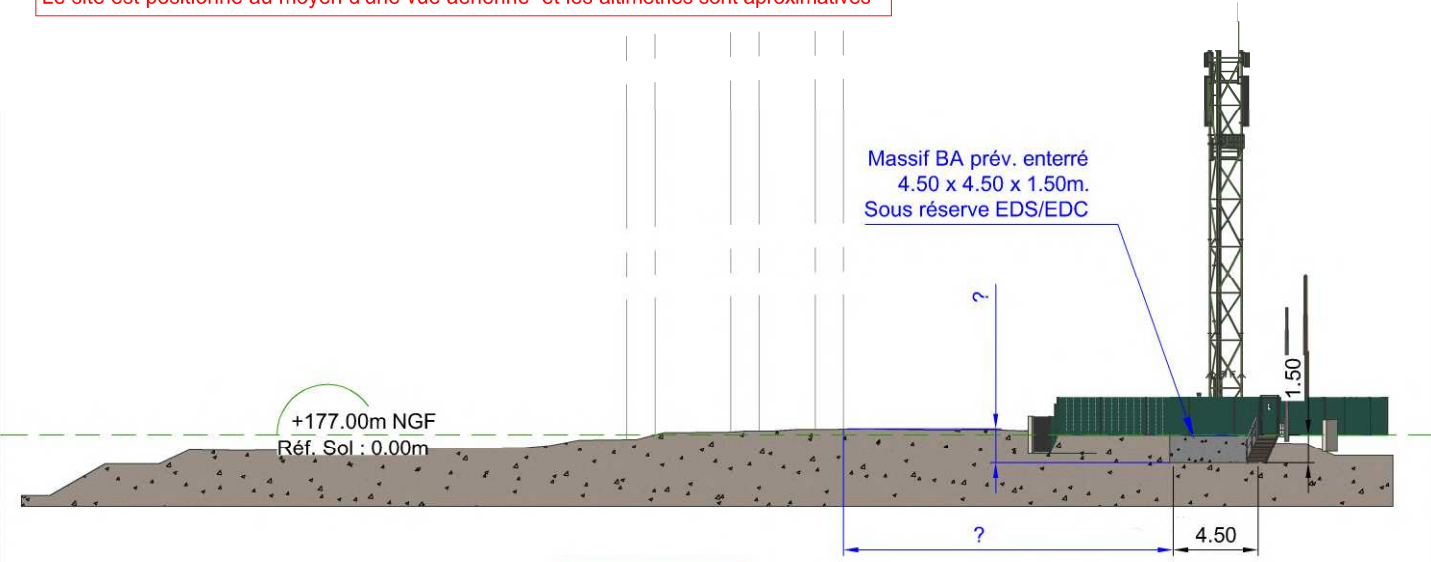
Plan de coupe A-A
